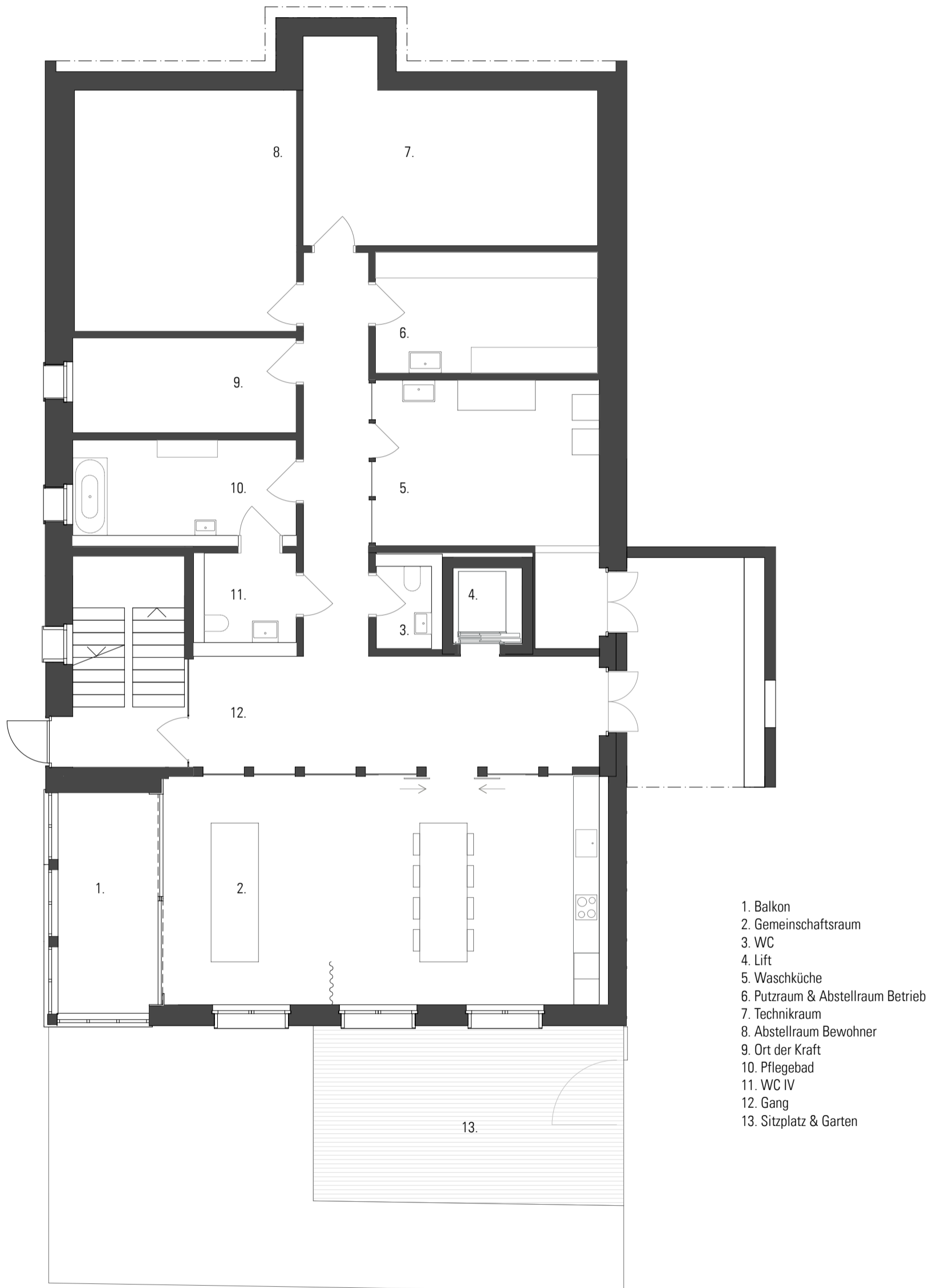
Grundriss EG
