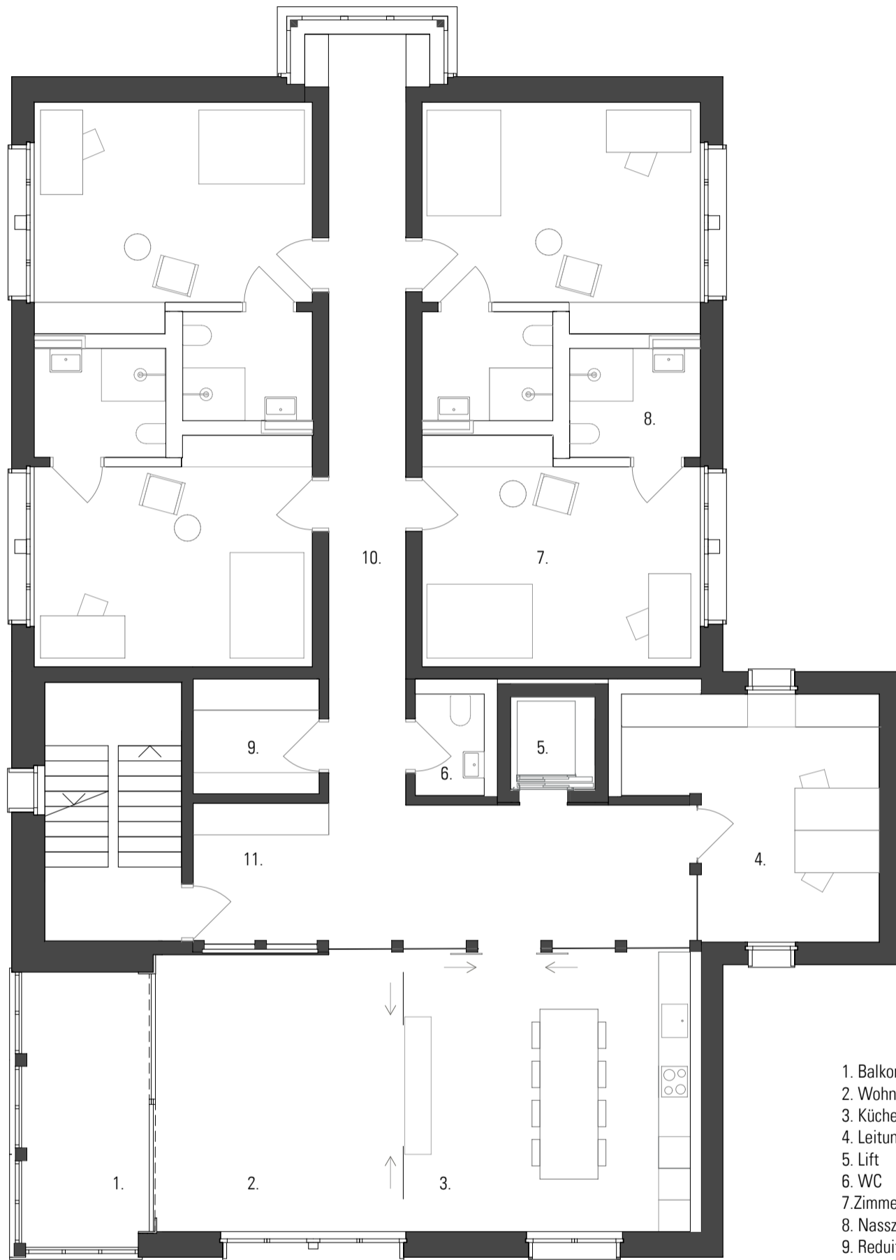
Grundriss 1.OG
