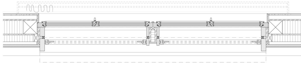
Grundriss
