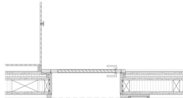
Grundriss
