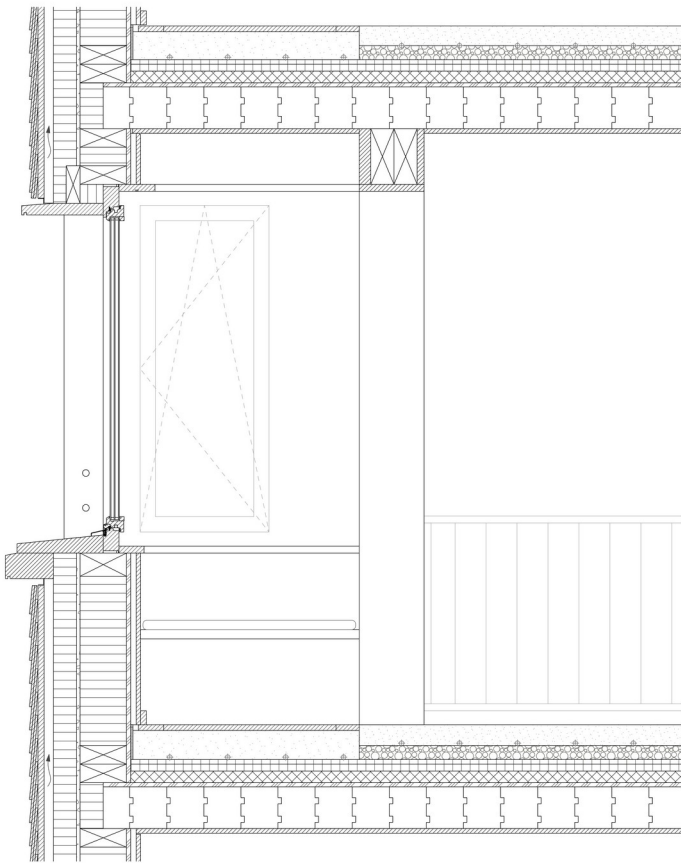
Schnitt
