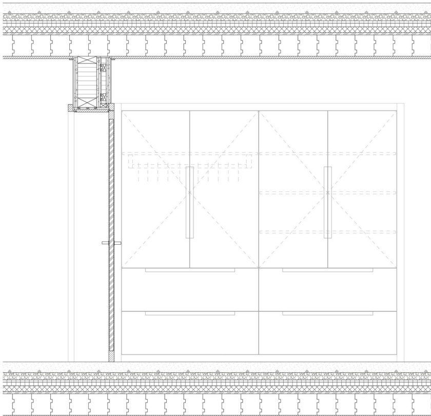
Schnitt
