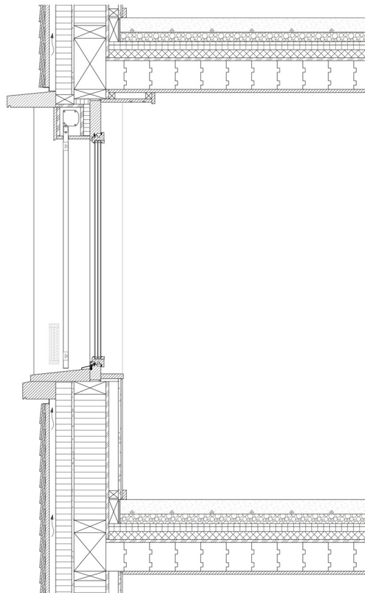
Schnitt
